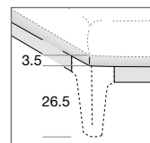
GIROLETTO LEGNO E IMBOTTITO WOODEN BED SURROUND AND UPHOLSTERED BLOCKBOARD
